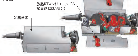
ノートPCアダプターの内部のイメージ
