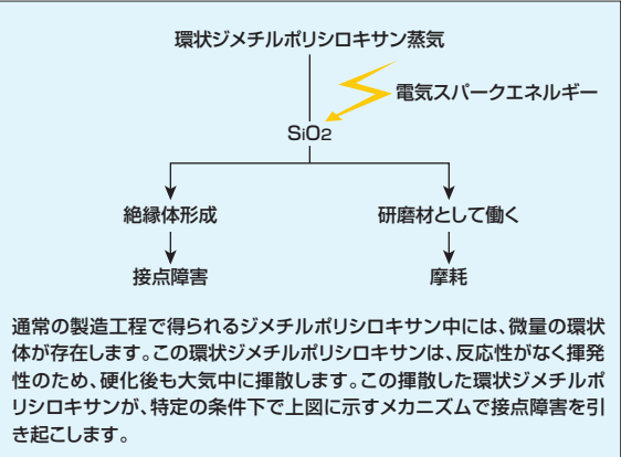
接点障害発生メカニズム
