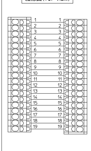
結線図 (TOP VIEW)
