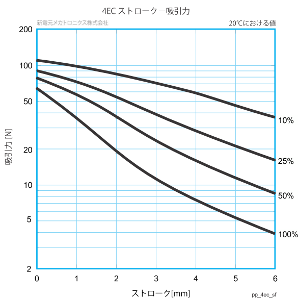
図表 4 4EC ストローク吸引力
