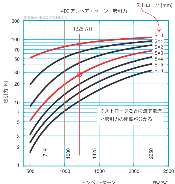
図表 2 4EC アンペア・ターン-吸引力
