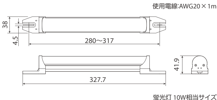
外形概略寸法図
