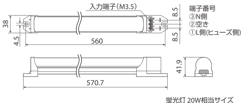
外形概略寸法図
