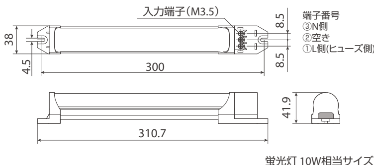
外形概略寸法図
