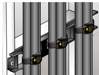
エンドレスタイを併用した、太径幹線などの固定
